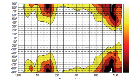
单只水平指向 Horizontal dispersion (-6dB) : 120°
