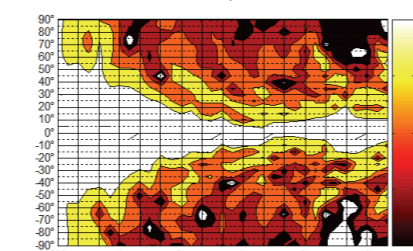
单只垂直指向 Vertical dispersion (-6dB) : 16°
